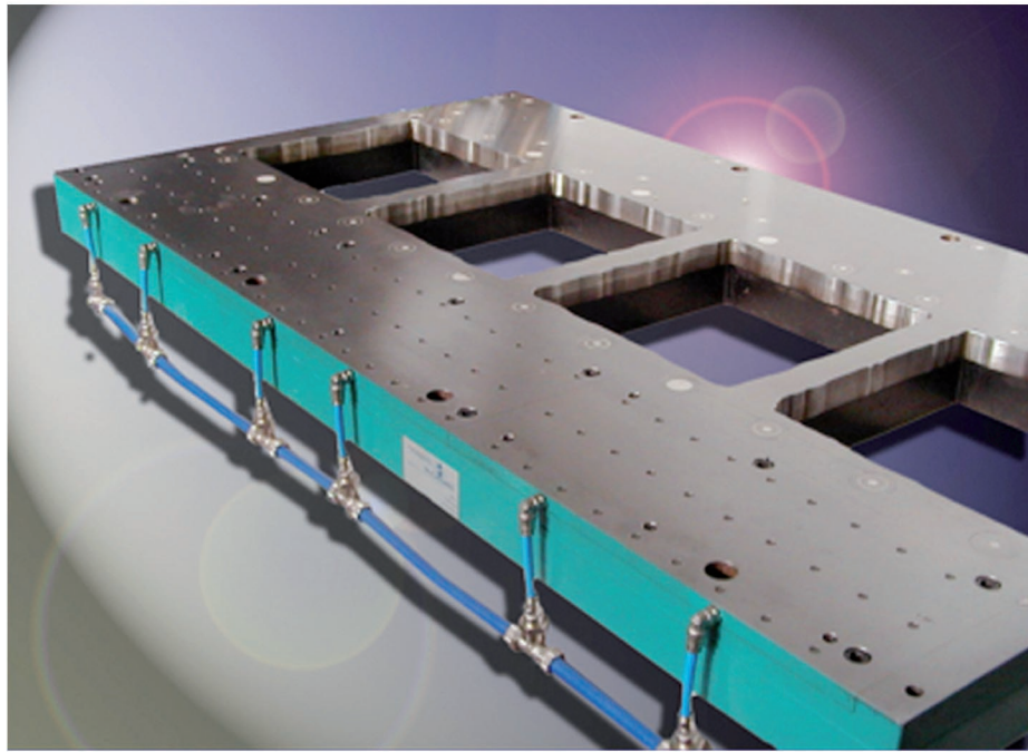
OVERCRAFT dispositivo pneumatico per la protezione della parte bella della piastrina in fase di estrazione Pneumatic device for the protection of tile good side, during the extraction phase
