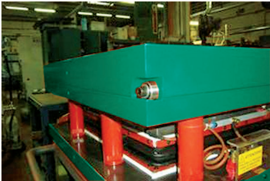
Stampo rientrante con matrice sfilabile, particolare Entry mould with removable cavity plate, detail
